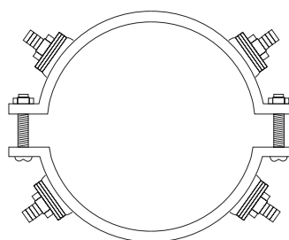
Type F Quatre borniers aux extrémités
