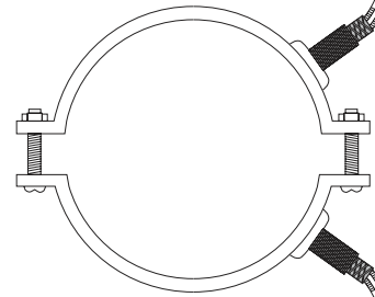
Type H Deux ressorts de chaque côté recouvrant fils avec tresse inox
